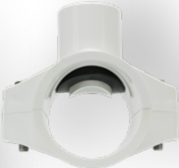
DIN Saddle Standard 63 mm Saddle
