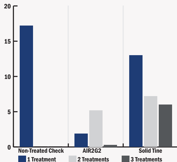
Surface Hardness (Gmax) 84 DAIT
